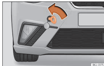
Fig. 78 Pare-chocs avant droit : œillet de remorquage.
