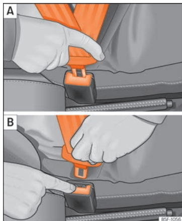
Fig. 94 Placer et retirer le pêne de verrouillage de la ceinture de sécurité.
