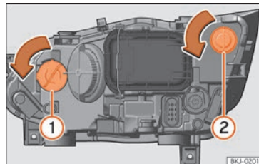
Fig. 106 Dans le compartiment moteur : ampoule du clignotant ① et ampoule du feu DRL (feu de circulation de jour) ②.
