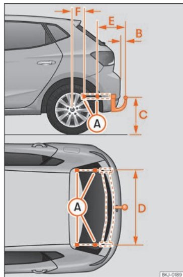
Fig. 264 Points de fixation du dispositif de remorquage.
