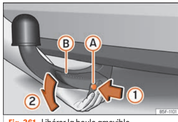
Fig. 261 Libérer la boule amovible
