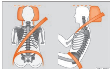
Fig. 19 Sangle de ceinture de sécurité bien ajustée et appuie-tête correctement réglé (vue de face et de côté)
