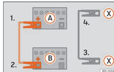
Fig. 81 Schéma de branchement pour les véhicules équipés du système Start-Stop.
