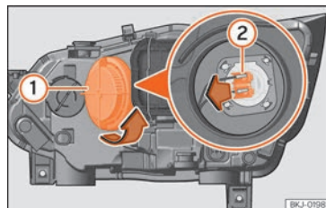
Fig. 103 Dans le compartiment moteur : ampoule des feux de route.
